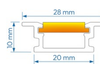
RAFD2010 COD: 7800591
