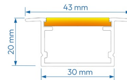
RAFD3020 COD: 7800587
