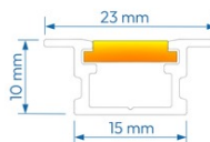
RAFD1510 COD: 7800589
