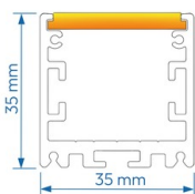
RFD3535 COD: 7800593
